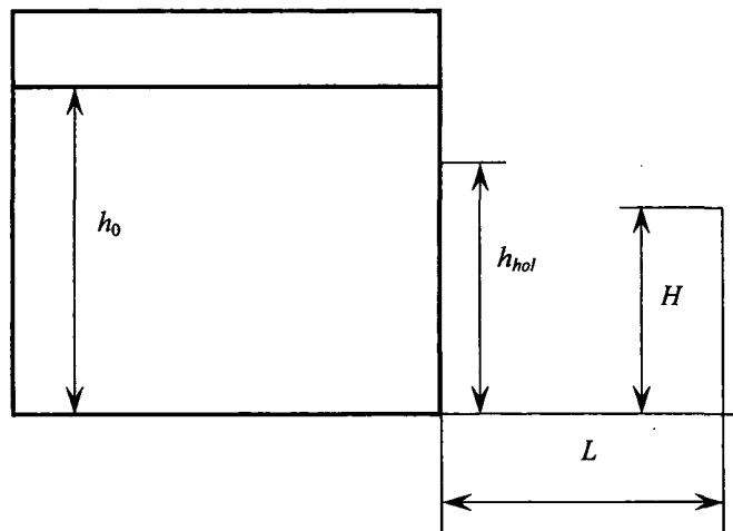
Рис. П3.1. Схема для расчета истечения жидкости из отверстия в резервуаре
